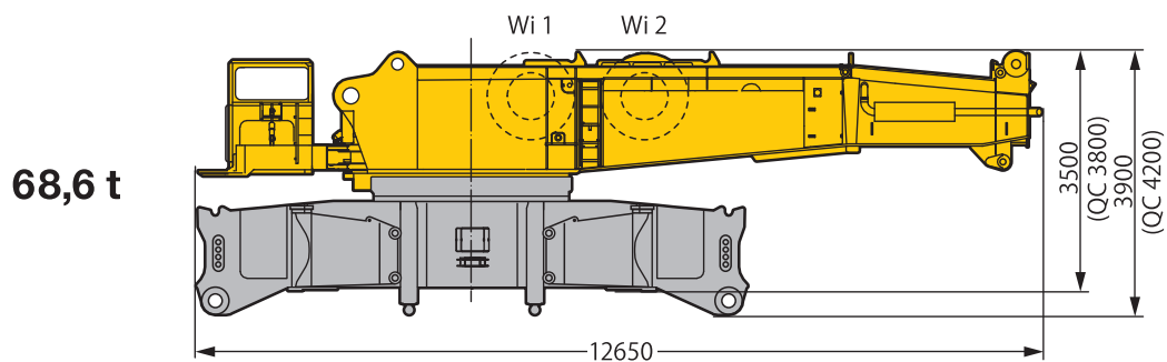
上部旋回体 & センターセクション & ウインチ1、2
