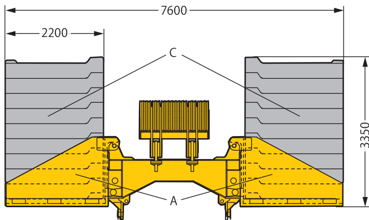
カウンターウェイト(上部旋回体上)
