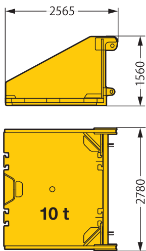
部材A
