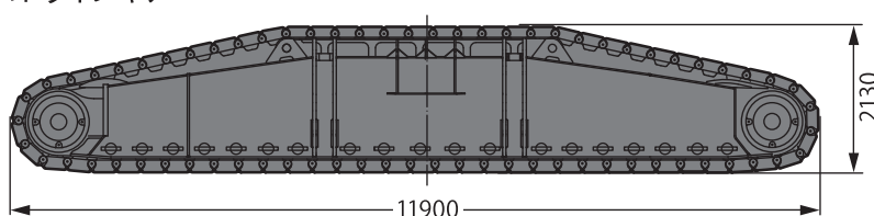
クローラシュー & 1ドライブギア
