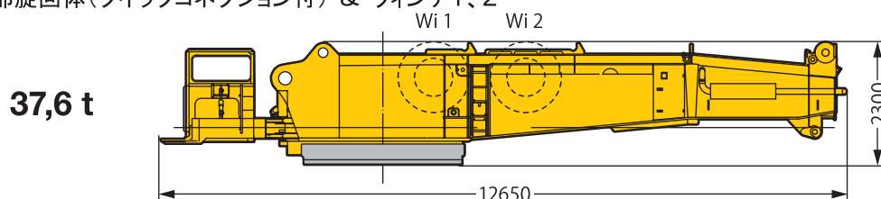
上部旋回体(クイックコネクション付) & ウインチ1、2
