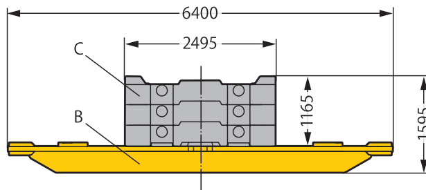
センターウェイト
